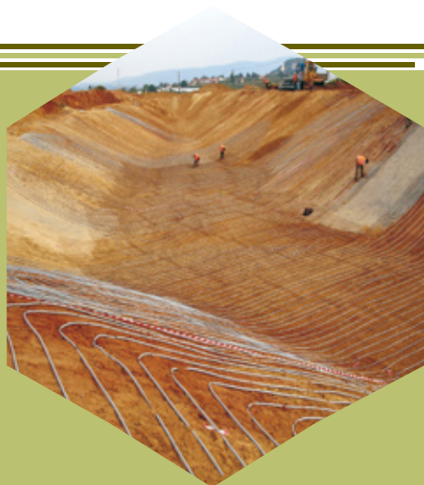
Ανανεώσιμες Πηγές Ενέργειας - Γεωθερμία: Άποψη του έργου Navarino Resorts - Dunes
